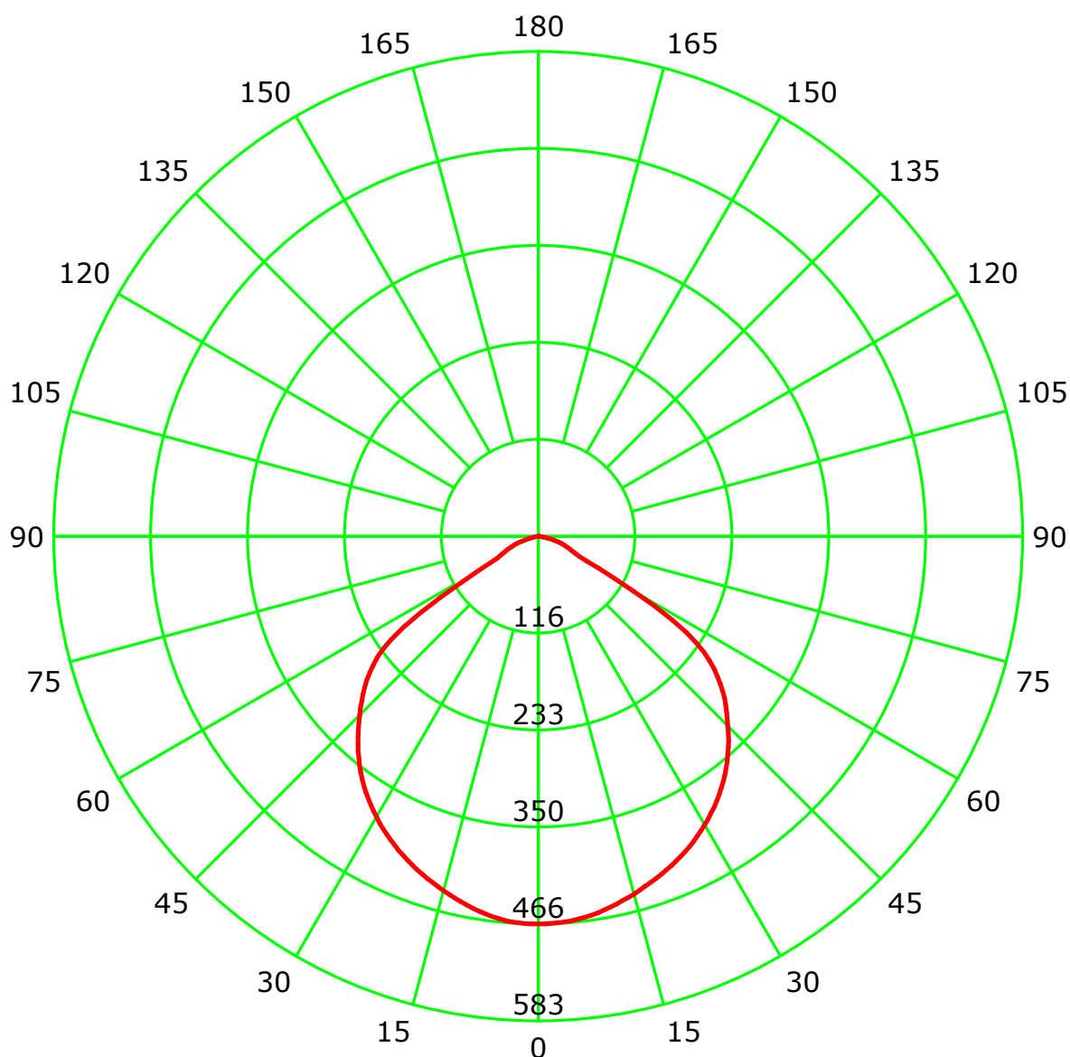
CURVA DE DISTRIBUCIÓN DE INTENSIDAD LUMINOSA (CD/KLM)
